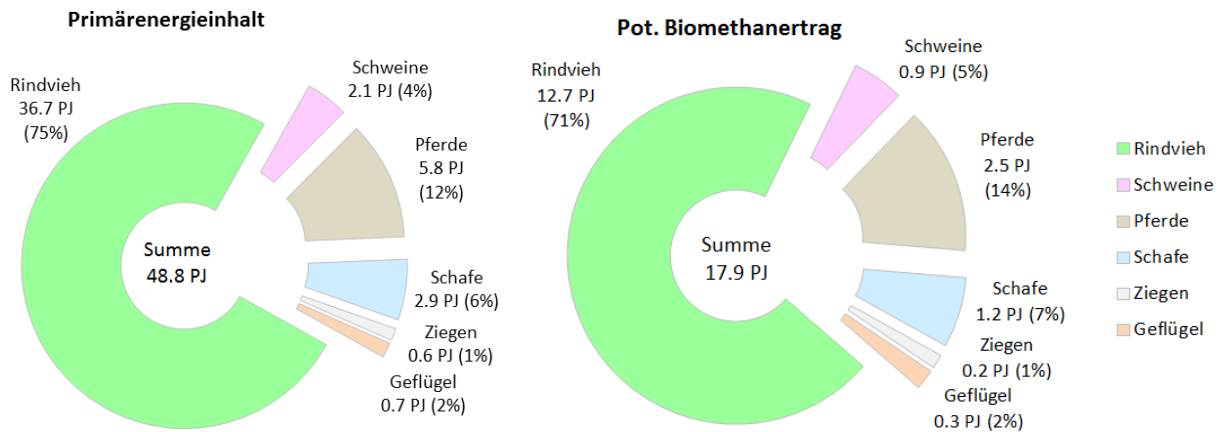
Abbildung 10: Theoretisches Potenzial, Hofdünger aus der landwirtschaftlichen Nutztierhaltung in der Schweiz, Primärenergieinhalt und potenzieller Biomethanertrag (Petajoule pro Jahr).
