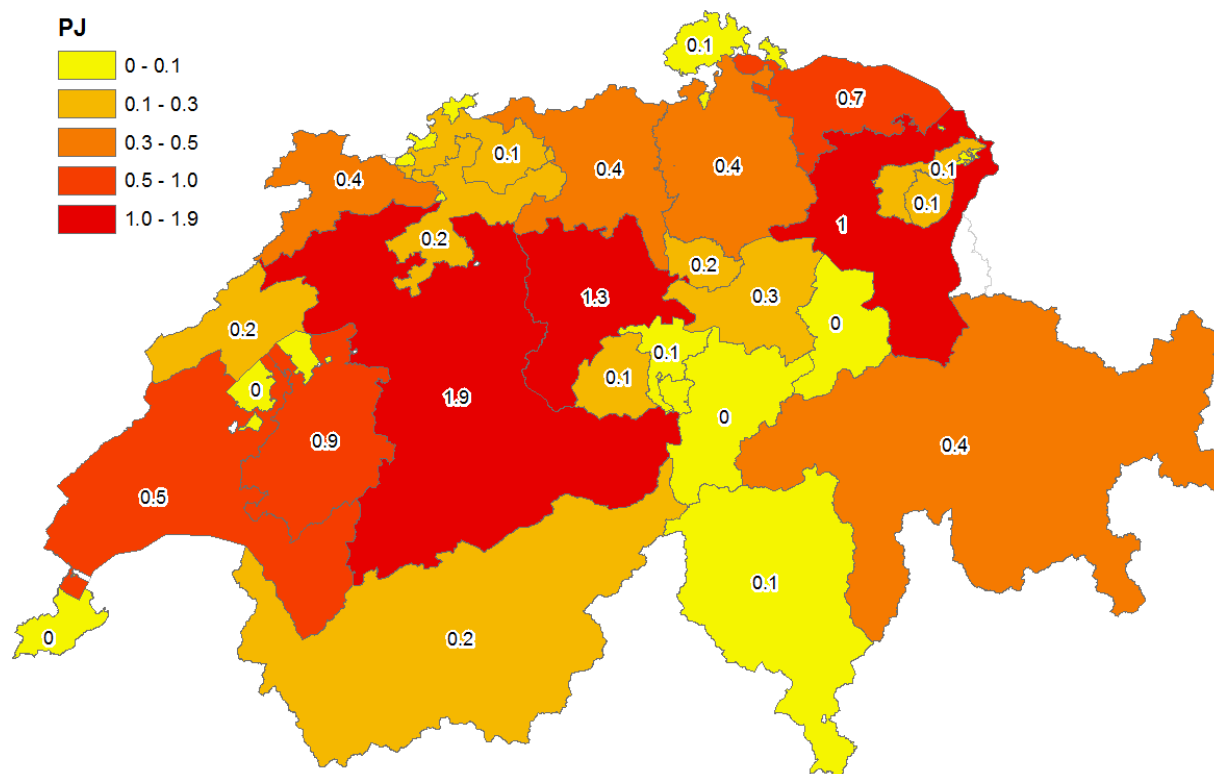
Abbildung 16: Nachhaltiges Potenzial (Abzug von Verlusten durch Weidegang und Gebieten mit zu geringem Hofdüngeranfall), kantonale Verteilung des potenziellen Biomethanertrags des Hofdüngers aus der landwirtschaftlichen Nutztierhaltung in der Schweiz (Petajoule pro Jahr).
