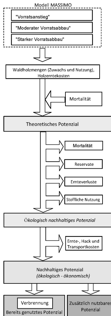
Abbildung 1: Übersicht zur Berechnung der Waldenergieholzpotenziale.
