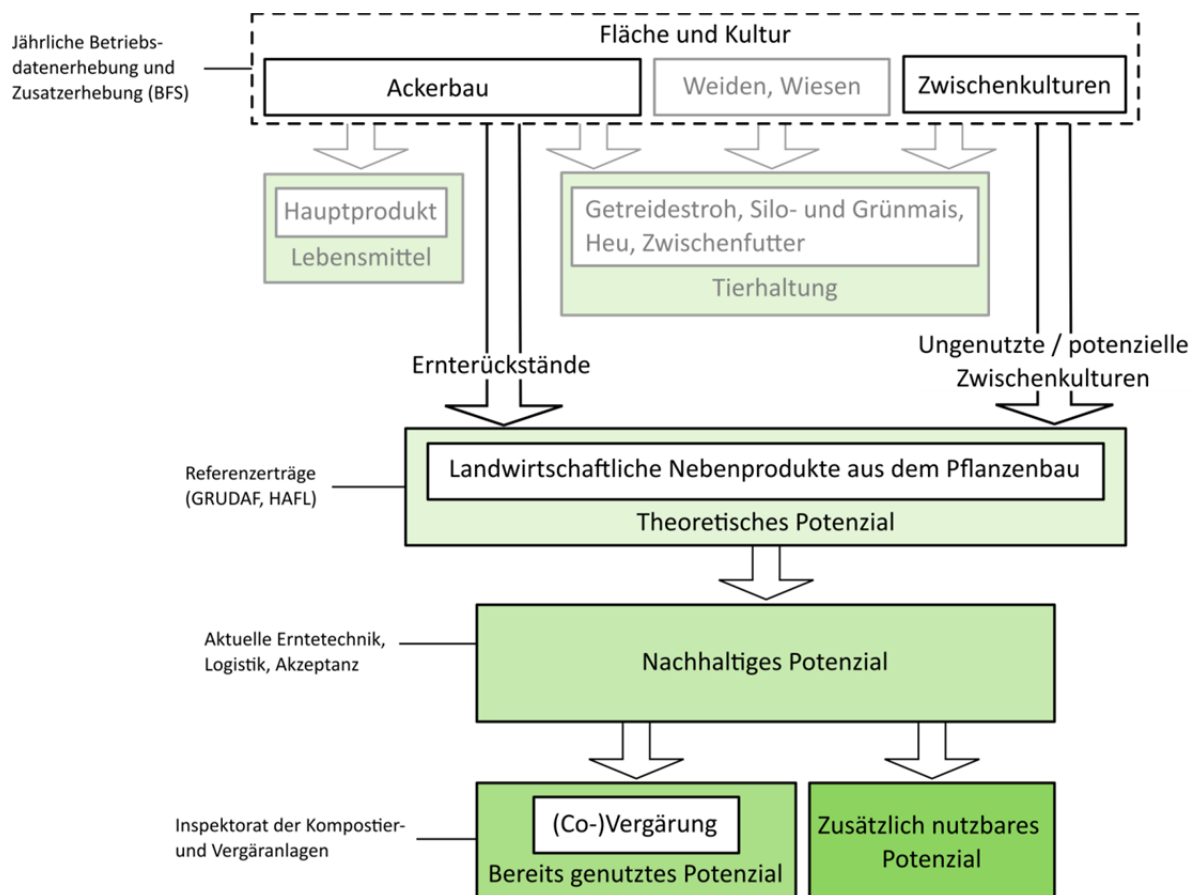
Abbildung 2: Modellansatz zur Ermittlung der energetischen Potenziale von landw. Nebenprodukten aus dem Pflanzenbau der Schweiz.
