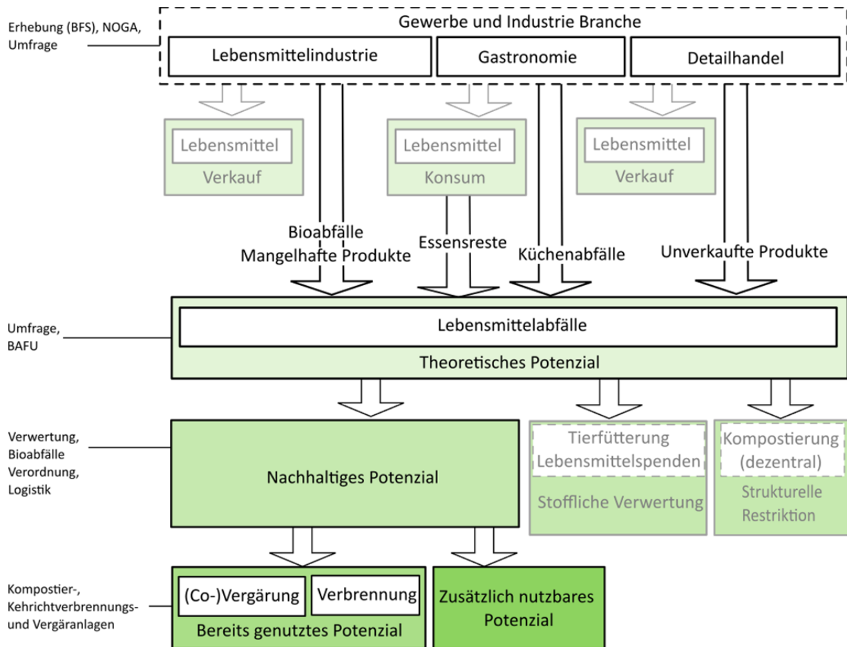
Abbildung 2: Modellansatz zur Ermittlung der energetischen Potenziale (Lebensmittelindustrie und -gewerbe).
