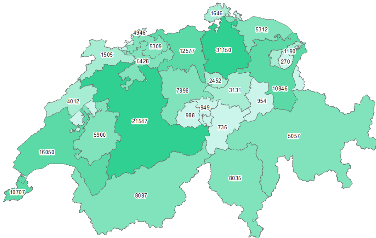
Abbildung 6: Theoretisches Potenzial, Menge Bio-Abfälle im Hauskehricht auf kantonaler Ebene (Tonnen Trockensubstanz pro Jahr).
