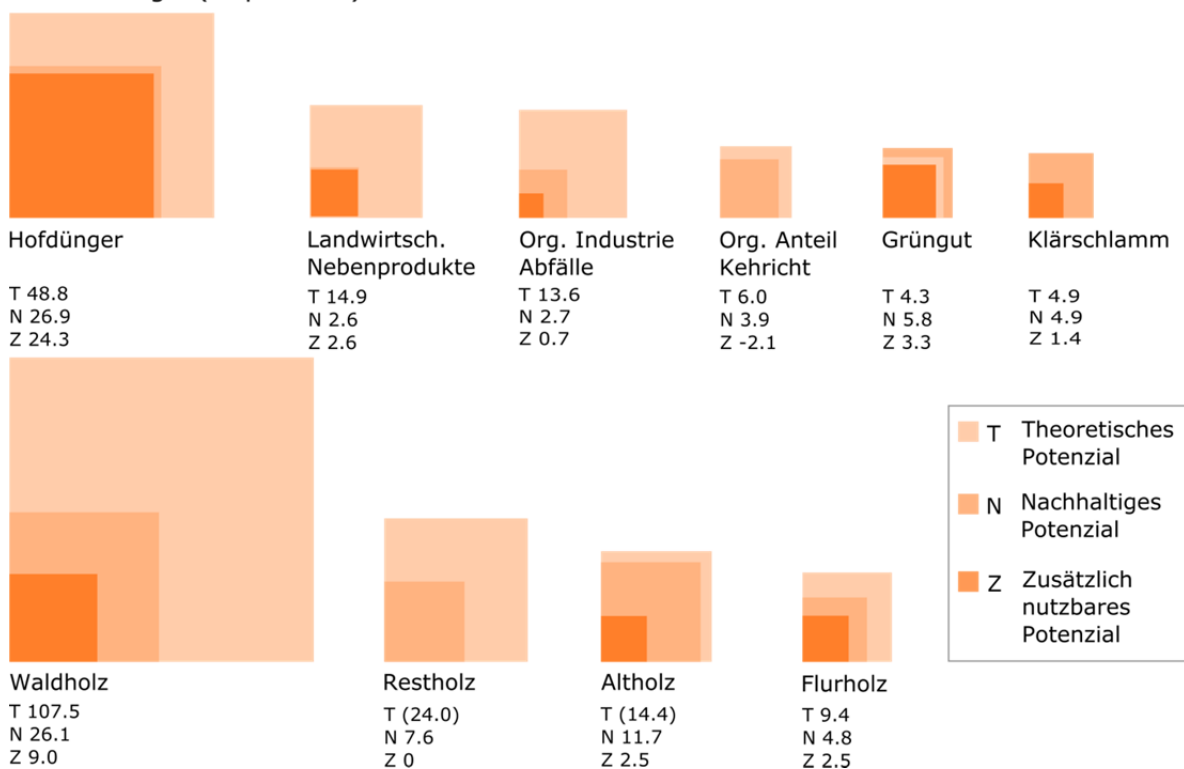
Abbildung 3: Primärenergiepotenziale aller 10 Biomassen in Petajoule (PJ) pro Jahr.
