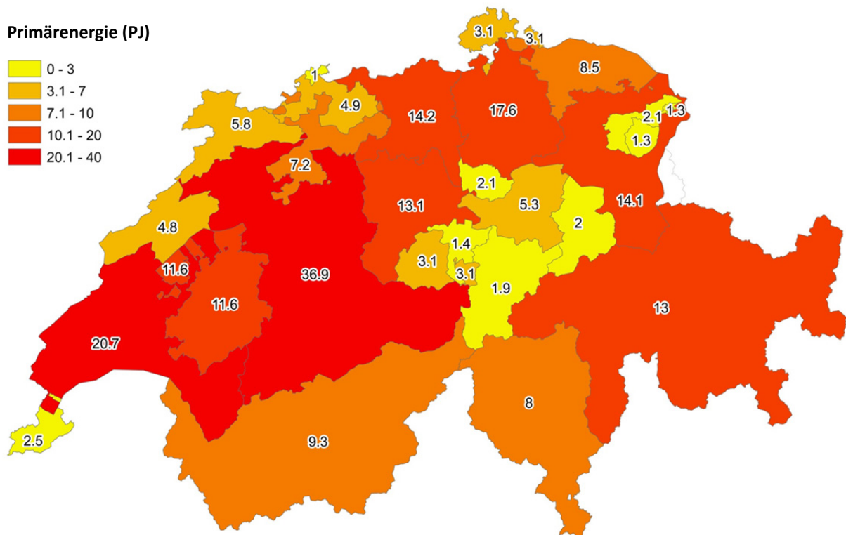
Abbildung 4: Räumliche Verteilung des theoretischen Primärenergiepotenzias aller 10 Biomassen nach Kantonen in Petajoule (PJ) pro Jahr.
