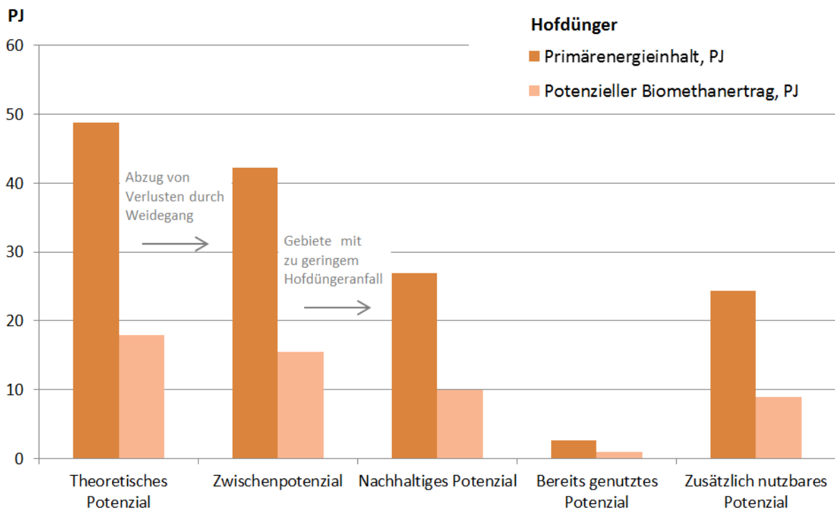
Abbildung 18: Potenzialanalyse des Hofdüngers aus der landwirtschaftlichen Nutztierhaltung der Schweiz.
