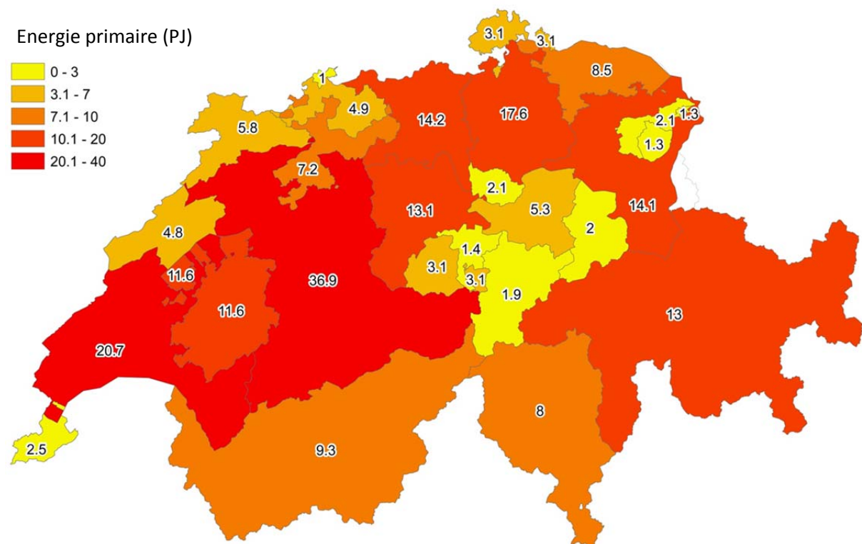
Figure 4: Répartition du potentiel en énergie primaire des 10 biomasses en pétajoules (PJ) par an pour chaque canton.
