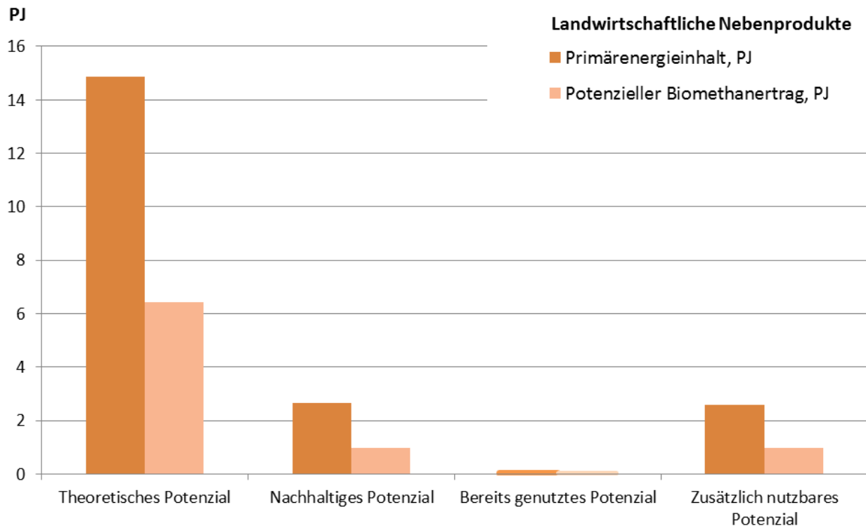
Abbildung 10: Potenzialanalyse der Energieinhalte der Nebenprodukte aus dem landw. Pflanzenbau in der Schweiz.
